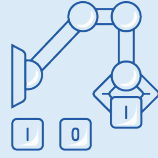
RPA
