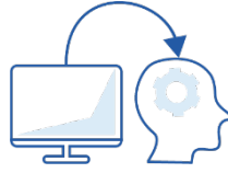
AI / ML
